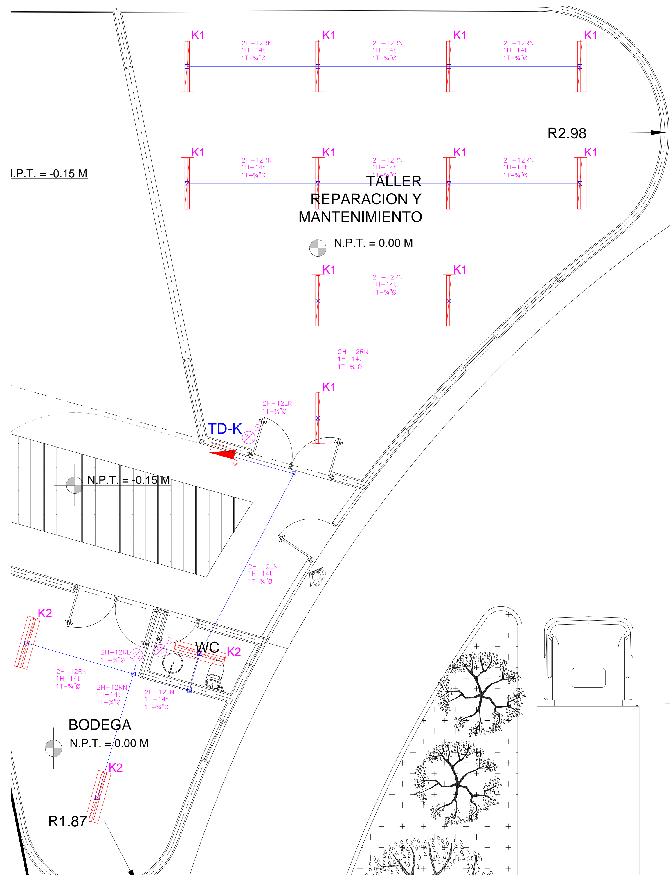
1 AREA DE MUELLE 1:50
