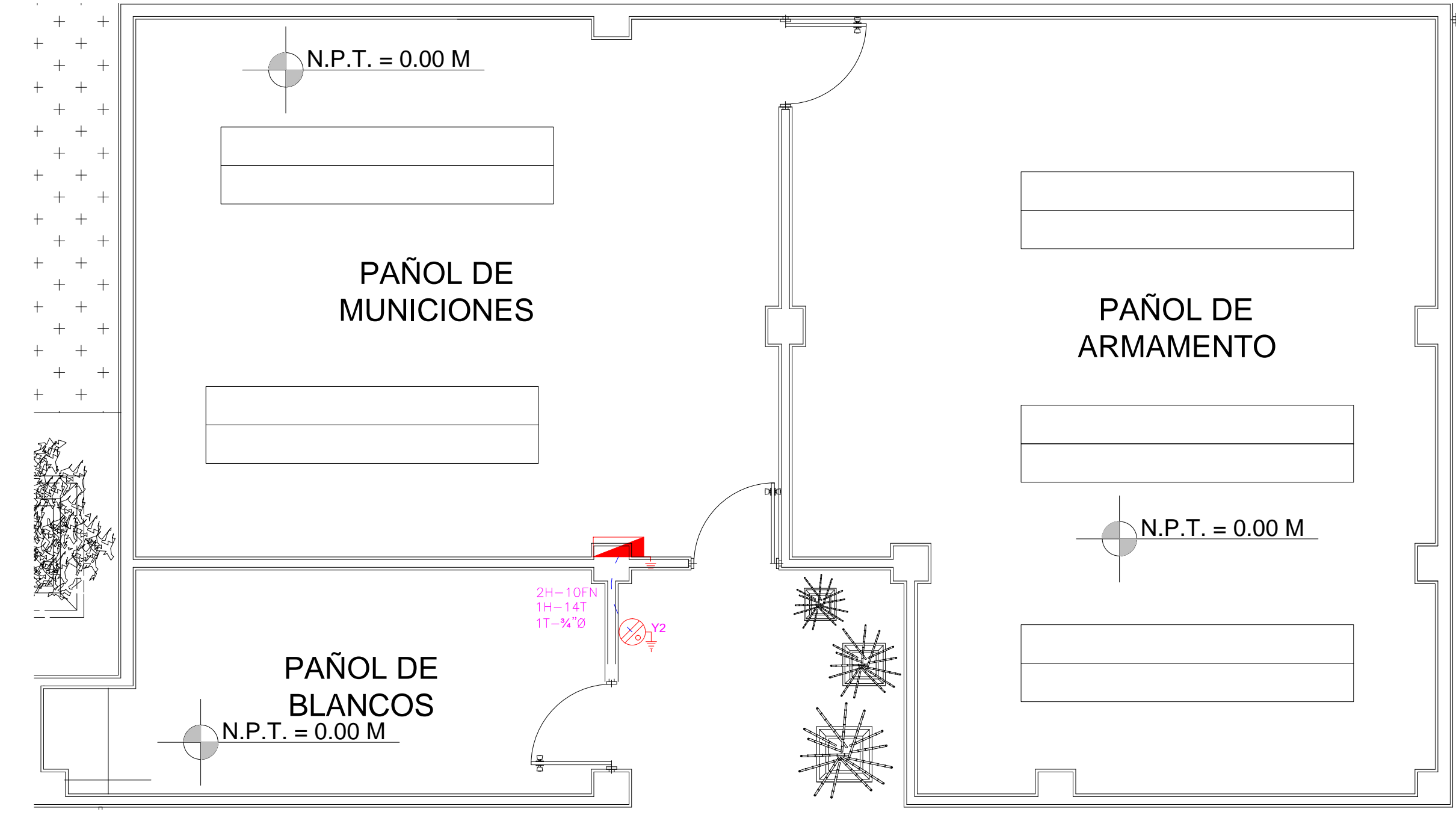
2 AREA DE PAÑOL DE MUNICIONES 1:50
