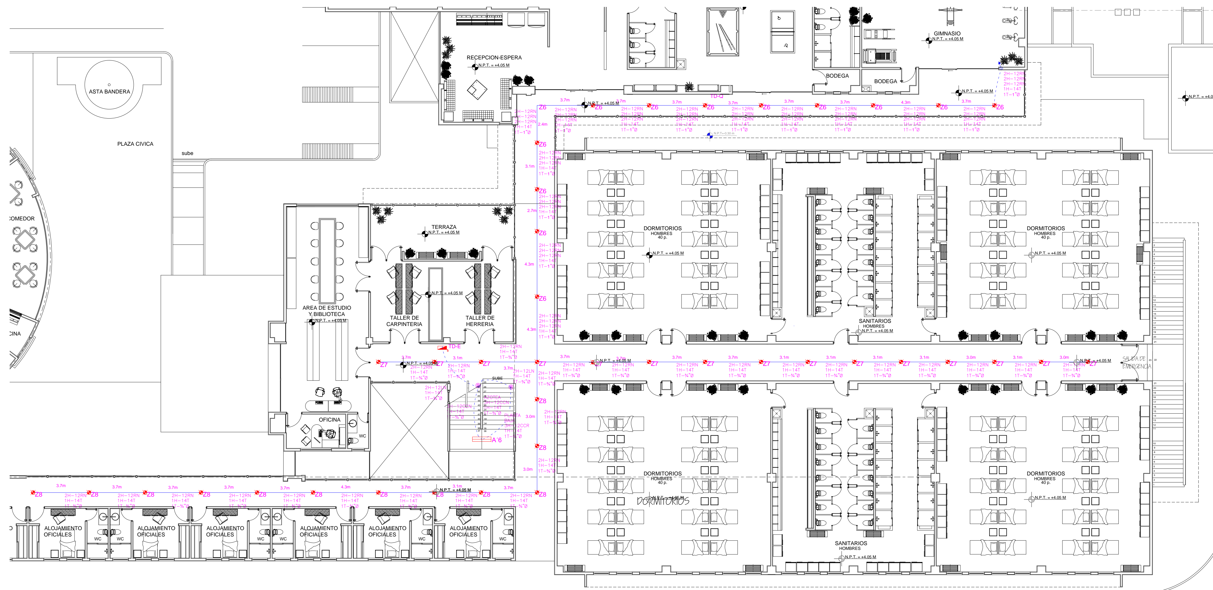
1 PASILLOS PLANTA PRIMER NIVEL 1:125
