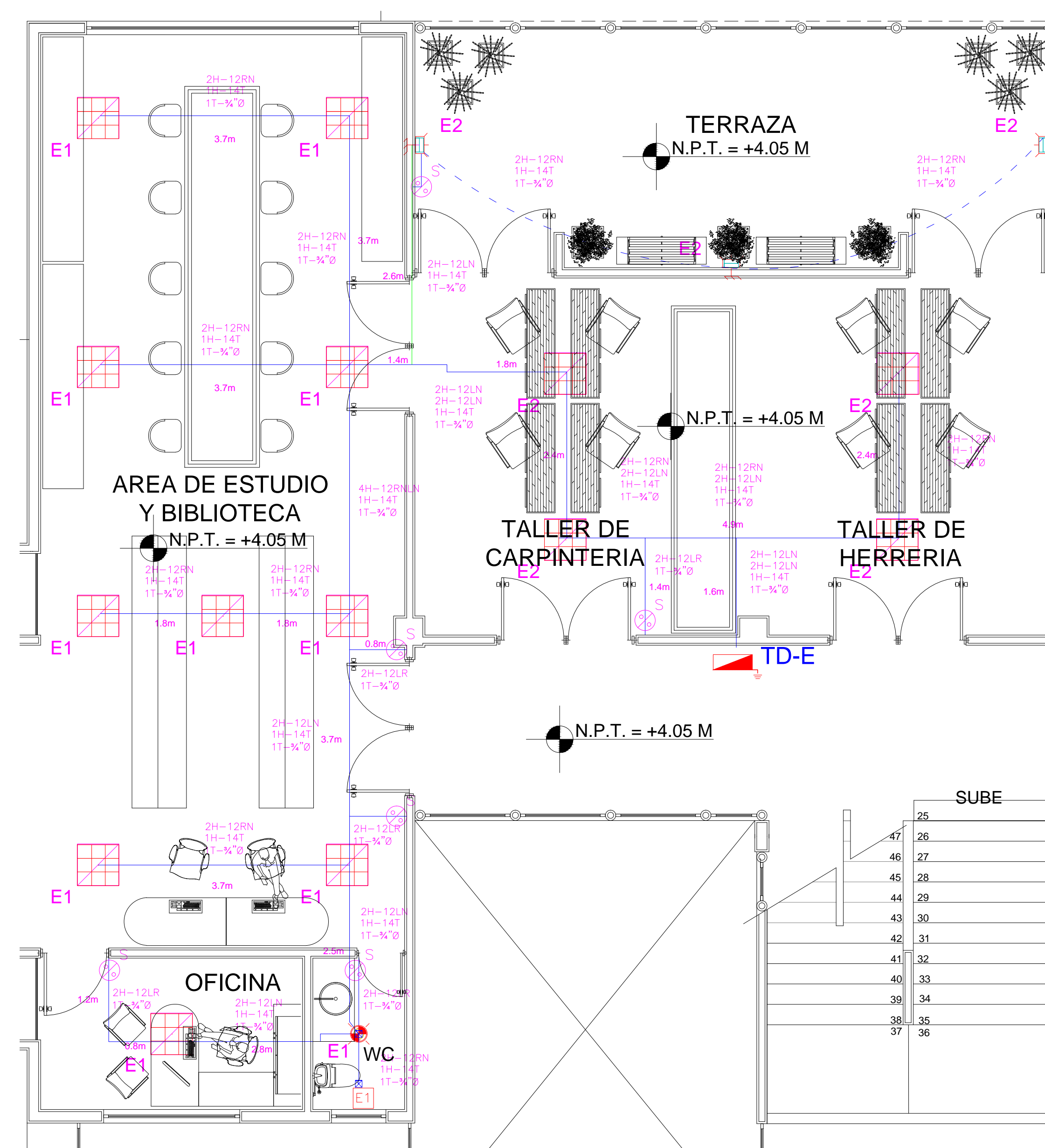
2 BIBLIOTECA Y TALLER DE CARPINTERIA 1:50
