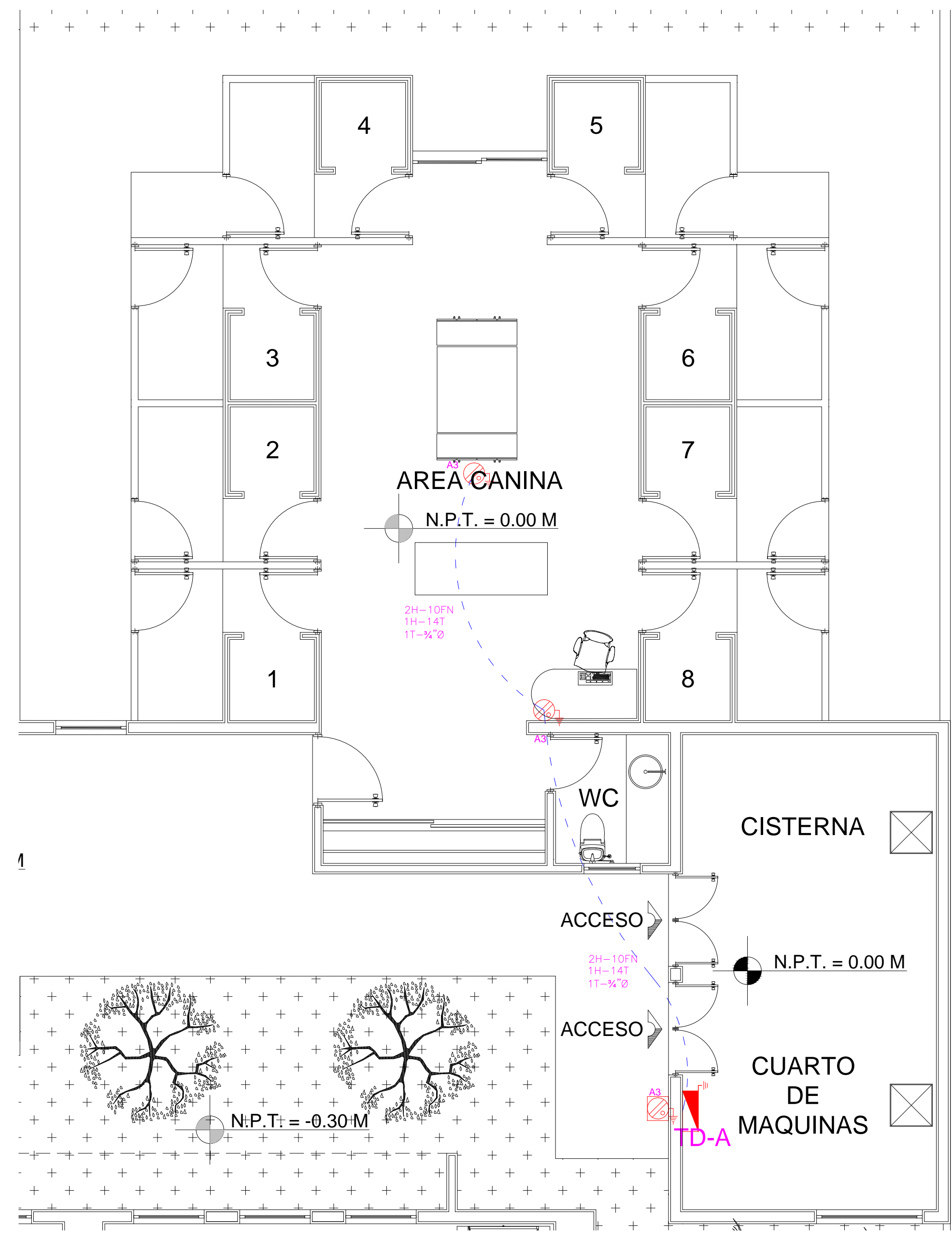
1 AREA CANINA 1:50
