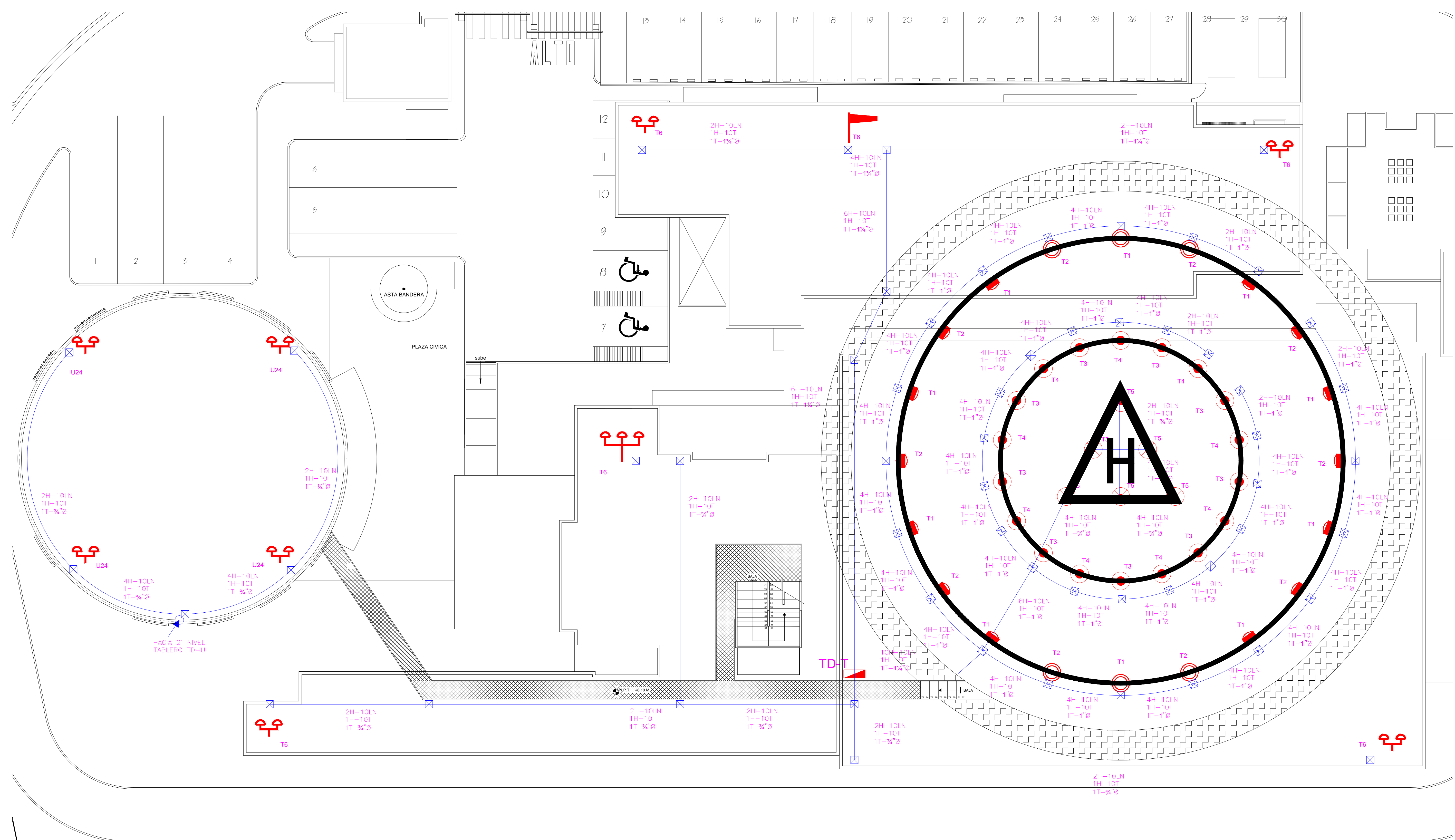
1 HELIPUERTO 1:125
