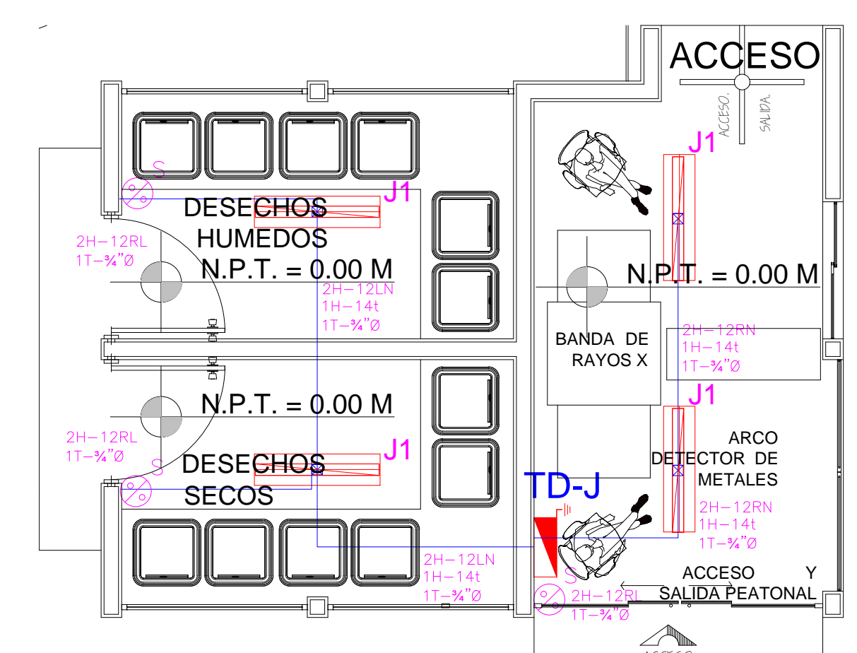
3 CASETA DE ACCESO 1:50
