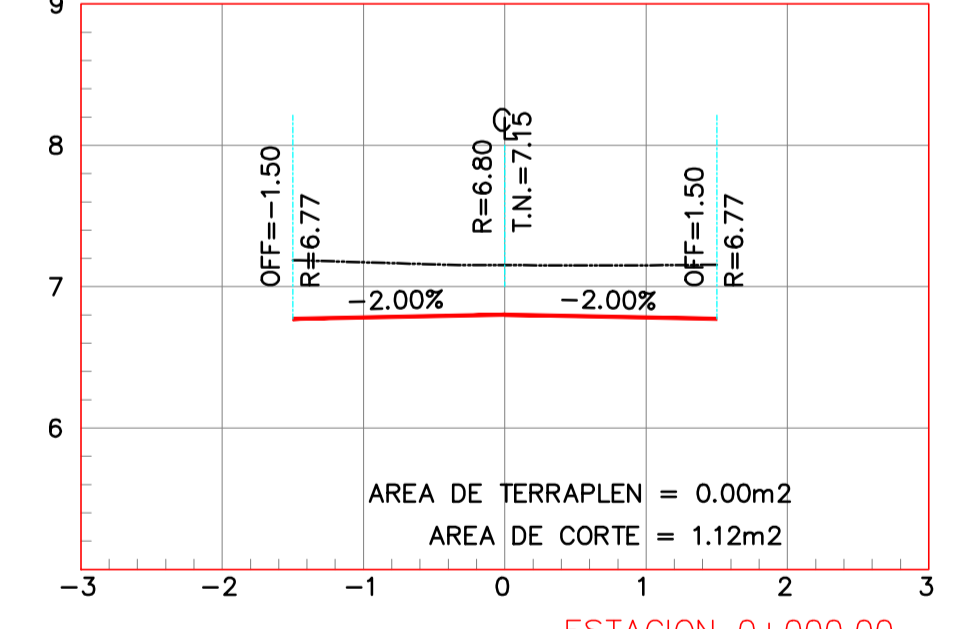
E S C A L A PLOTEO 1 : 100
