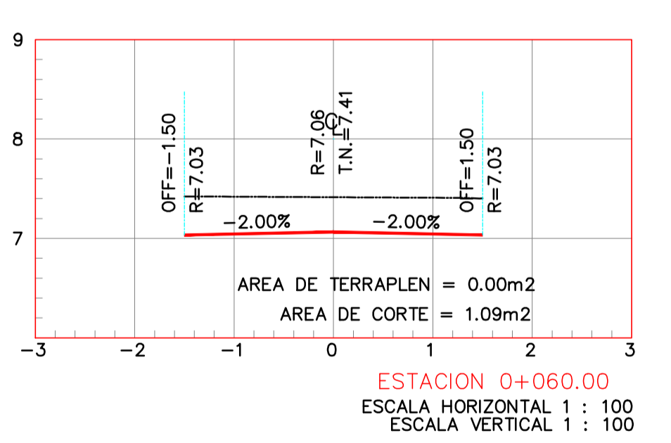
SECCIONES E S C A L A 1 : 100
