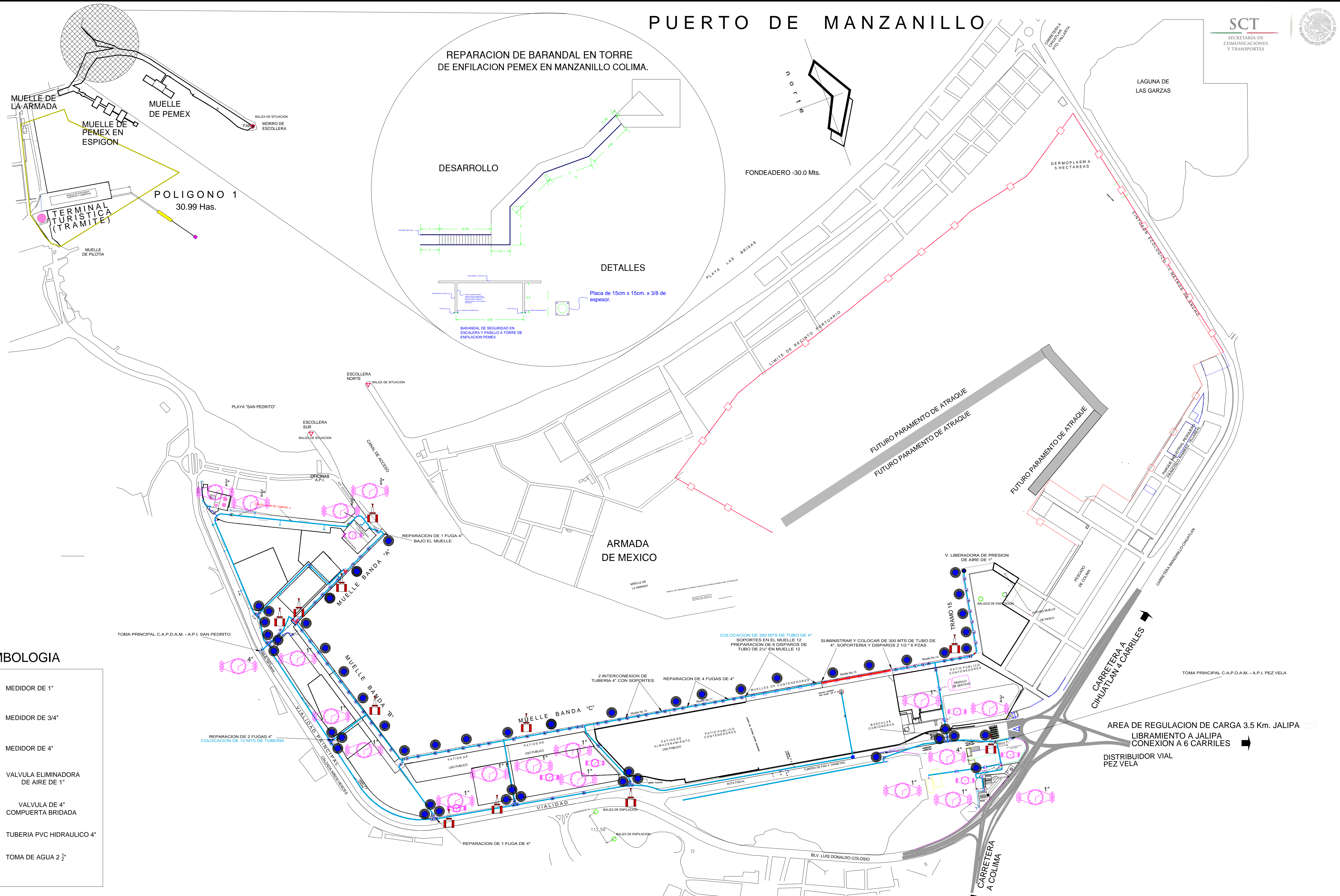
PLANO GENERAL DE LA RED HIDRAULICA EN EL PUERTO INTERIOR DE SAN PEDRITO MANZANILLO, COL.
