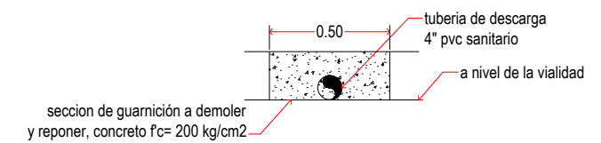
CORTE A-A
