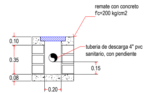
Registro a base de tabique castillos con armex 15-15 concreto f'c=200 kg/cm2
