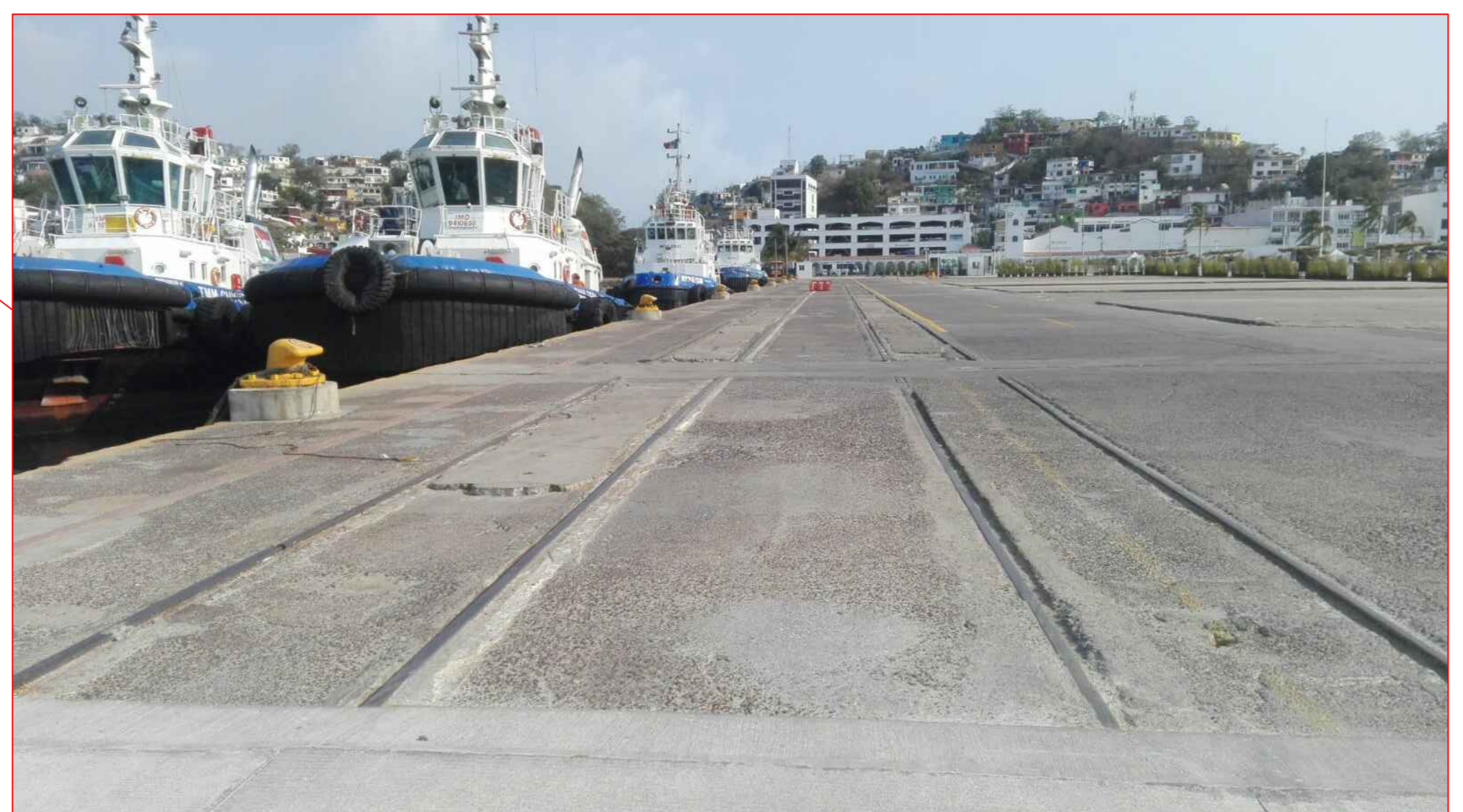
Reparación de losa de concreto area 9.24 \times 200m = 1,848.00 \text{ m}^2
