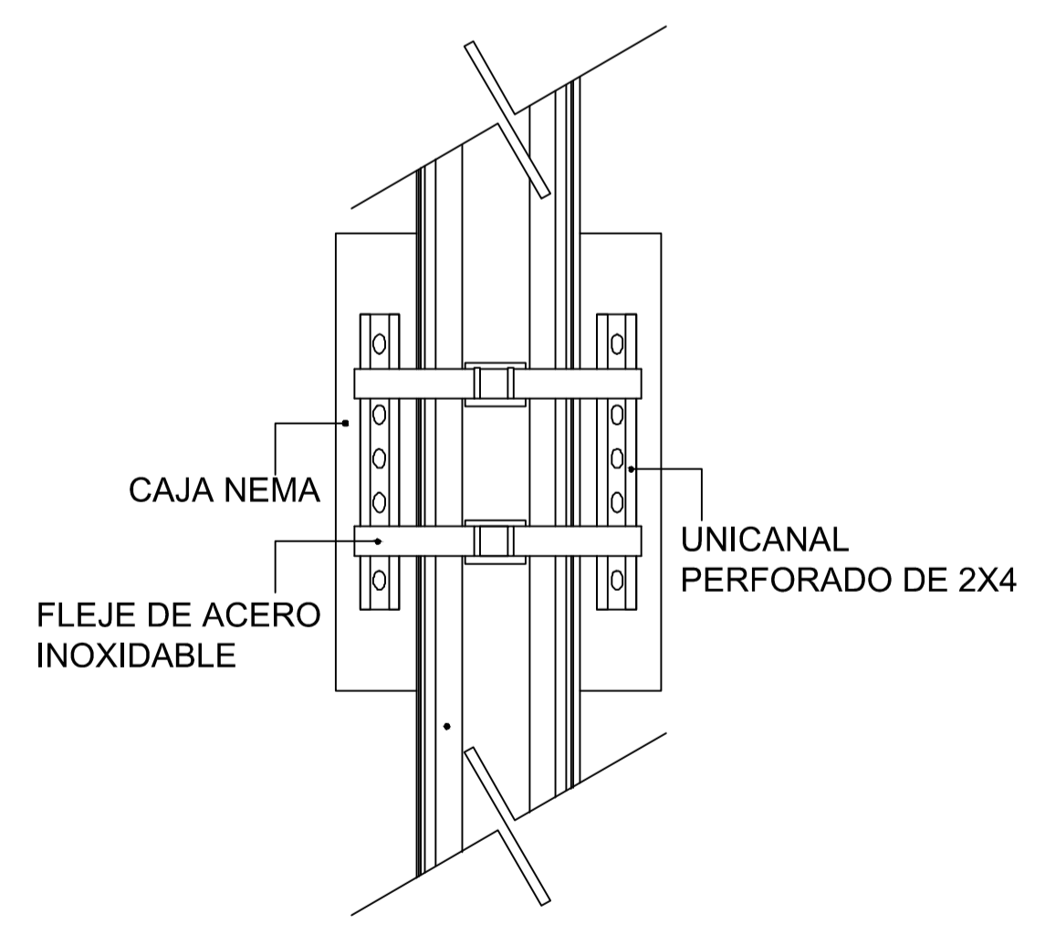
DETALLE DE COLOCACION Y FIJACION DE CAJA NEMA IP66 72X51X25 CM
